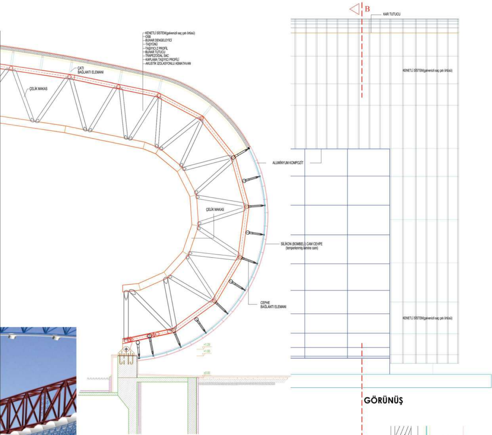
B-B KESİTİ
